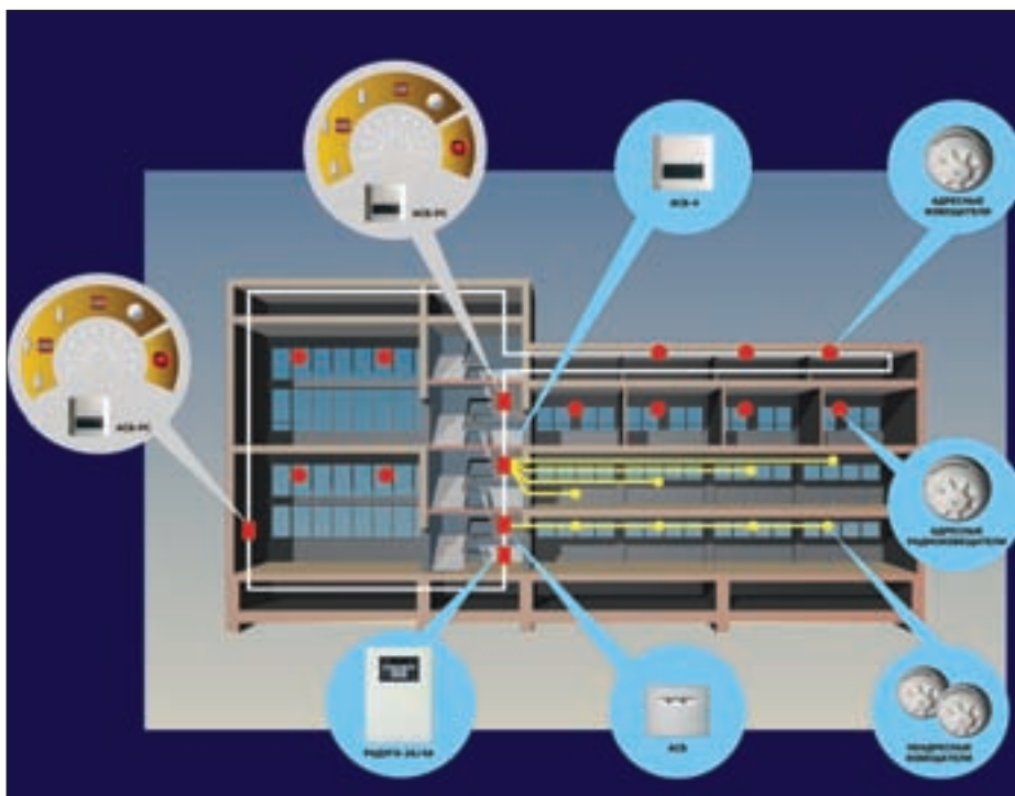
Рис. 4. Совместное использование проводной системы РАДУГА-2А/4А® и радиоканальной системы СТРЕЛЕЦ®
